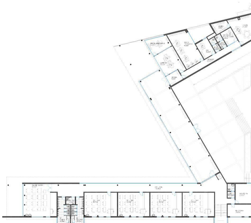
Imagem n.º II – Planta da Escola – Primeiro Andar
